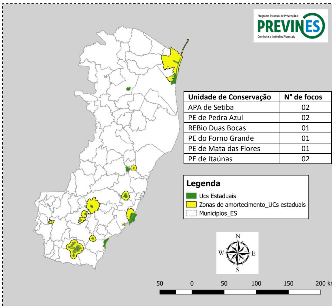
Figura 1: Unidades de Conservação estaduais com foco de incêndio registrado no período de janeiro a abril de 2018.
