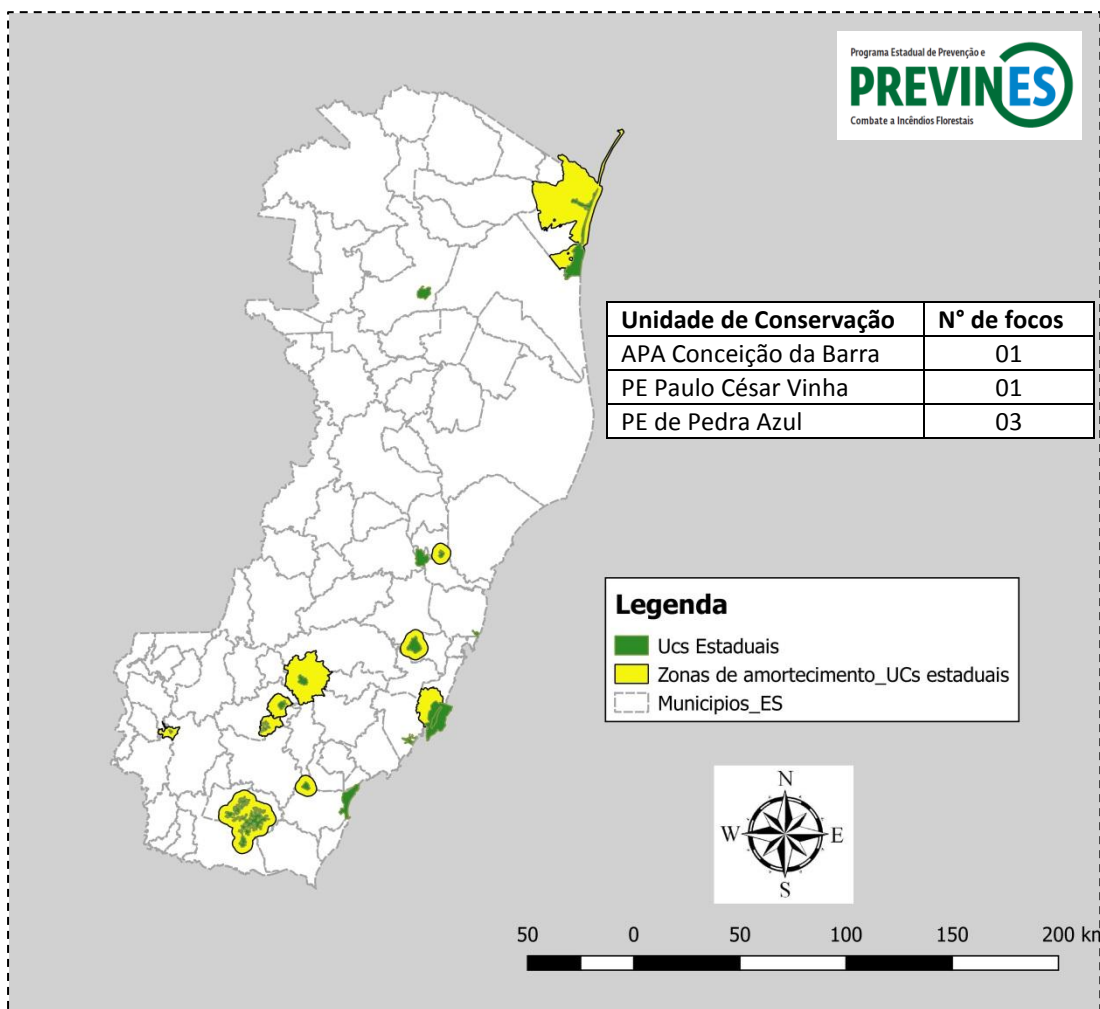
Figura 1: Unidades de Conservação estaduais com foco de incêndio registrado no período de 01/01/17 a 30/04/17.
